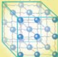
MOLECOLE DI UN SOLIDO
