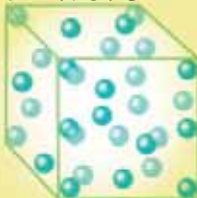
MOLECOLE DI UN GAS
